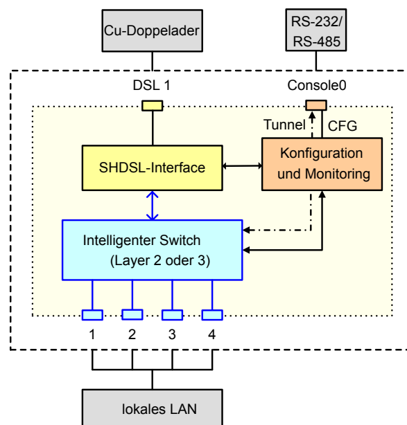
Abbildung 1: Prinzipschaltbild der Baugruppe 500NMD01
